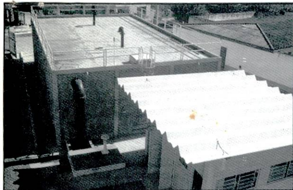
RESERVATÓRIO DA ETA 600 MIL LITROS
