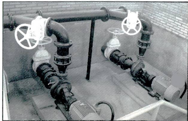
BOMBAS DE RECALQUE DA ETA
